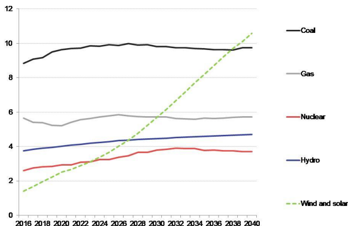
図：発電資源別電力生産の推移
